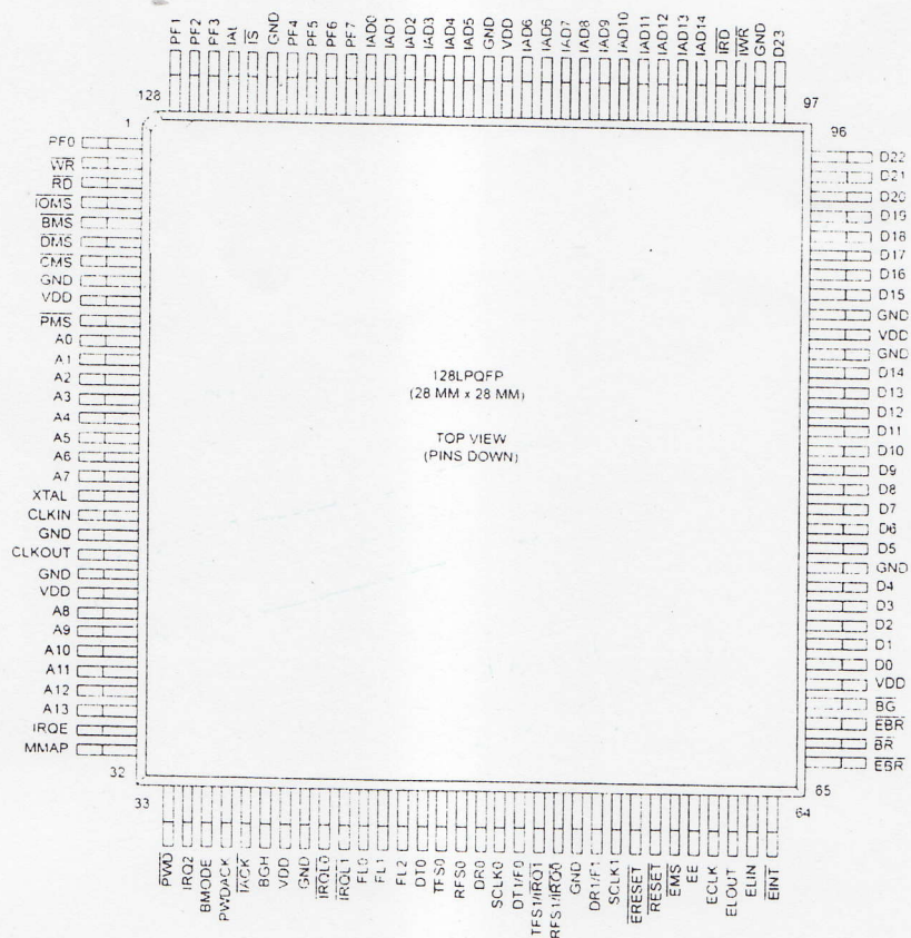
Вариант исполнения процессора в корпусе PQFP-128
